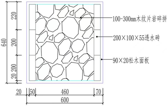
冰纹路游步道铺装平面图 图 5
