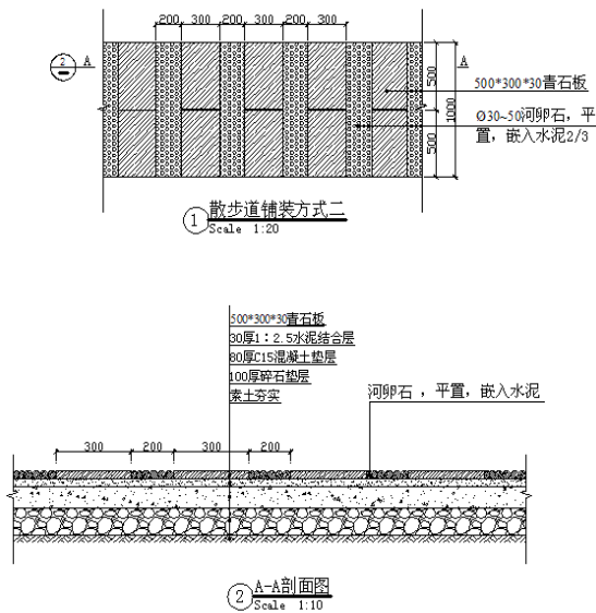
图 8-2 园路施工图
