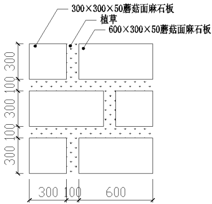
石板嵌草路（局部）平面图
