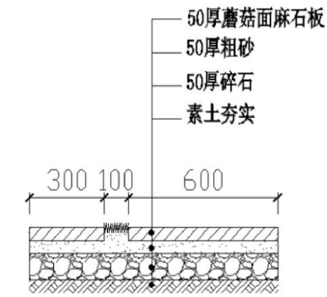
石板嵌草路剖面图
