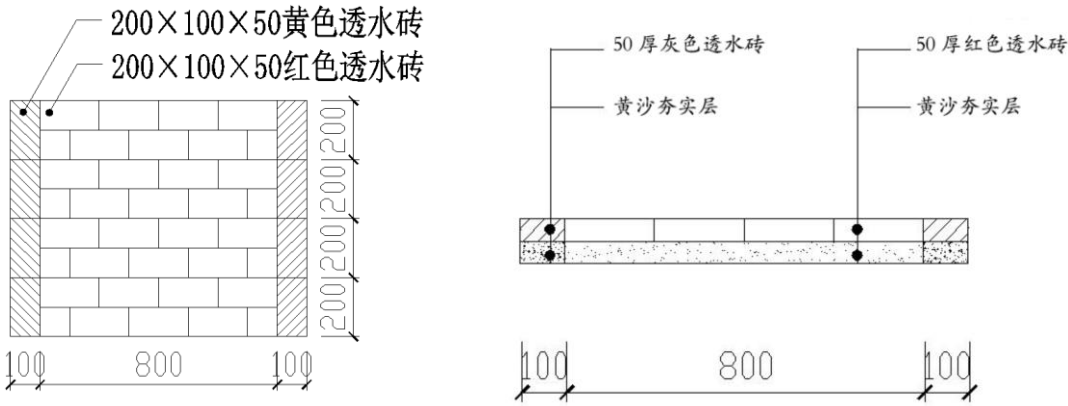
透水砖园路(局部)平面图
