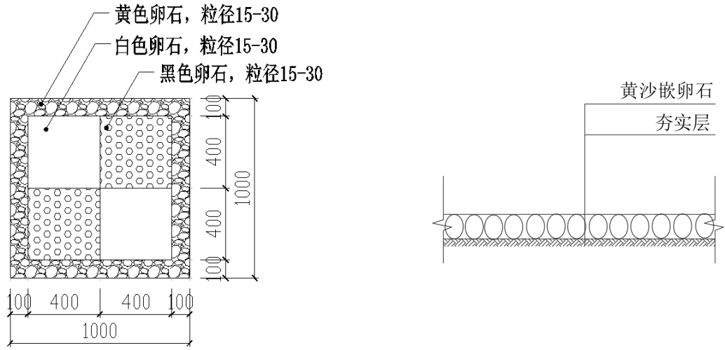
卵石路（局部）平面图
