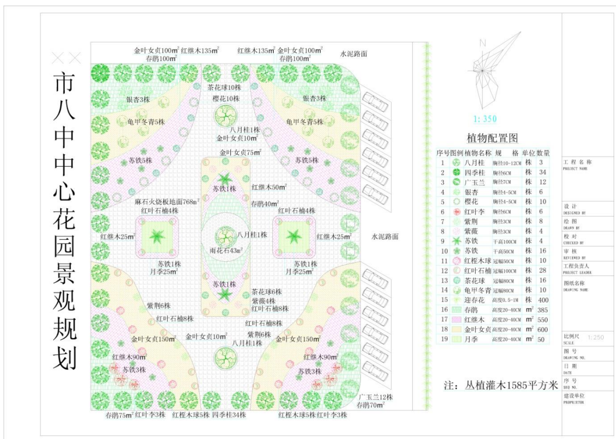
图 9-2 园林植物种植工程平面图
