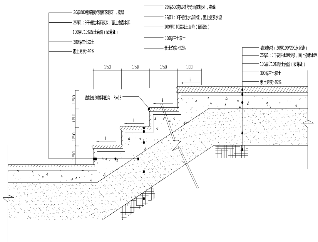
台阶断面详图
